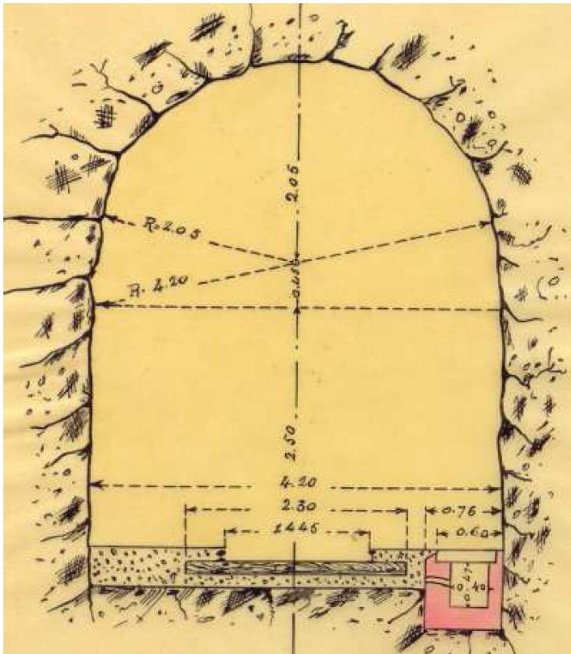
Sezione tipo delle gallerie estratta dal progetto di realizzazione della ferrovia lungo la Valle Brembana
